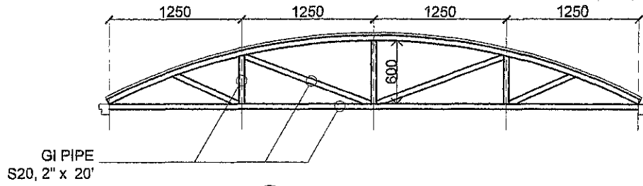
TRUSS DETAIL SCALE: 1: 50 mm
